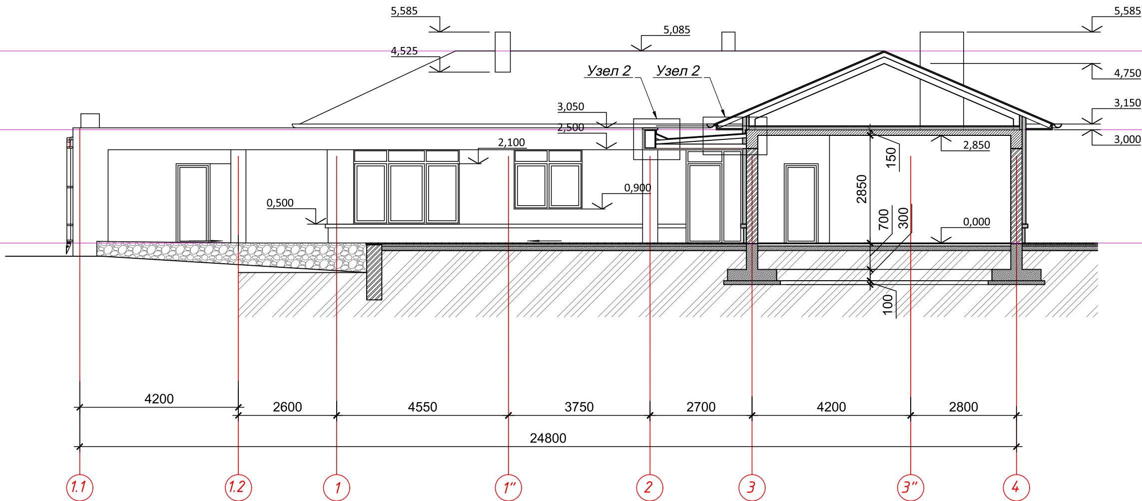
Разрез 5-5
