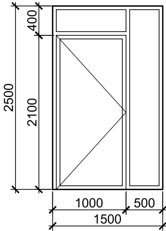
Д-1 Кол-во: 1шт
