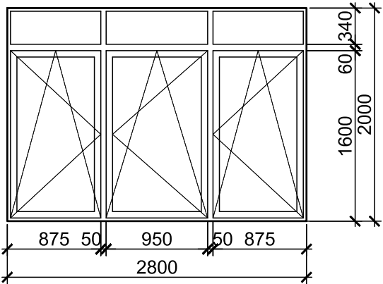
Позиция 3 Кол-во: 1шт
