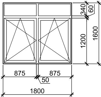
Позиция 5 Кол-во: 2шт
