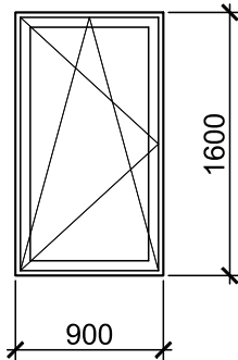
Позиция 5 Кол-во: 2шт
